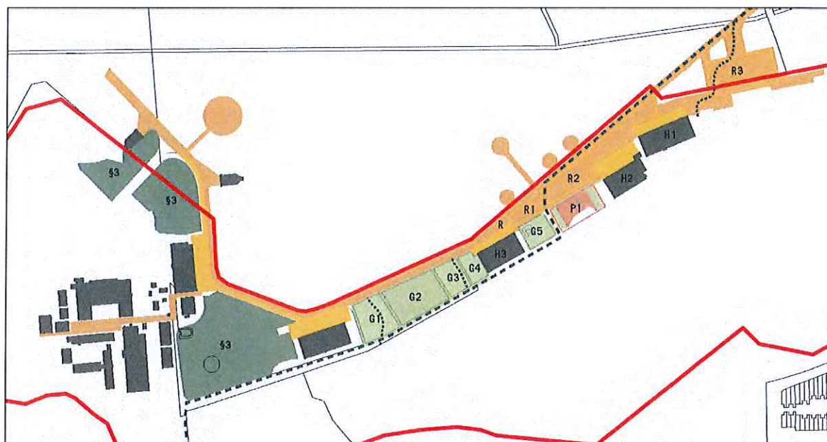
Tegning 10: Principiel disponering af rullearealerne nord for Hangar 1-4
